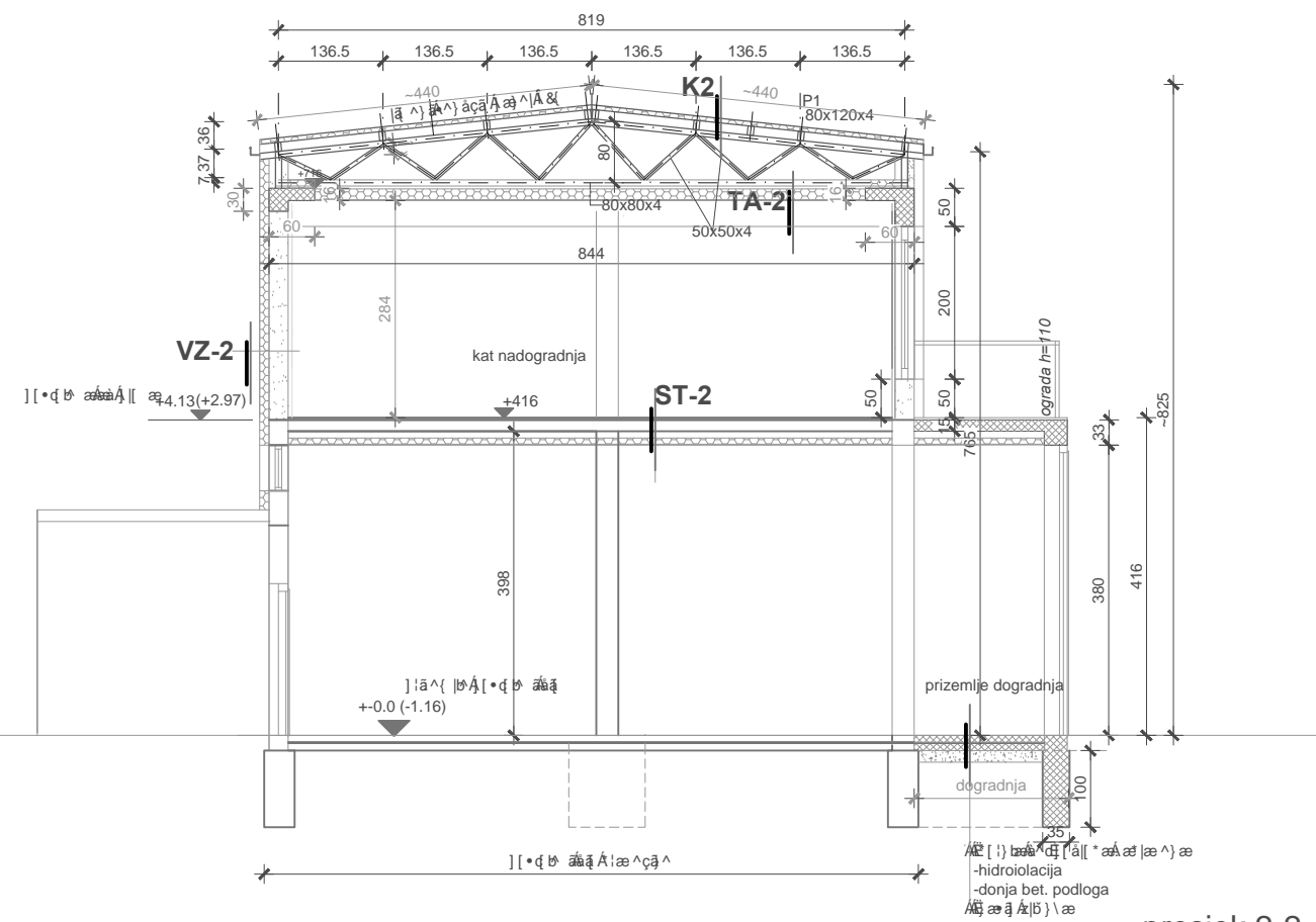
presjek 2-2
